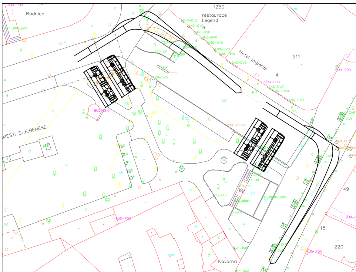
Obr. č. 1 – Interní orientační ověření vlečných křivek pro 15m autobus do technické mapy GISMO
