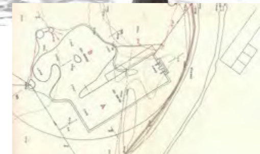
Půdorys koupaliště. A – bazén pro plavce se skokanskými můstkami, B – bazén pro neplavce a děti. Vpravo za řekou budouva čerpací stanice VZ, která stojí dodnes.
