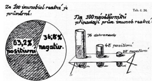
Statistické vyjádření počtu nemocných na 100 případů za rok 1930, tabulka z publikace Deset let činnosti Ústavu sociálně zdravotní péče lidové (dispensáře) MLPT Moravská Ostrava 1921–1931 (Moravská Ostrava, 1931).
