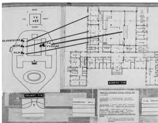
Situační náčrtek televizního střediska Ostrava (TVS), půdorys přízemí budovy TVS. Betonážní práce hlavní budovy byly zahájeny 1. dubna 1955.
